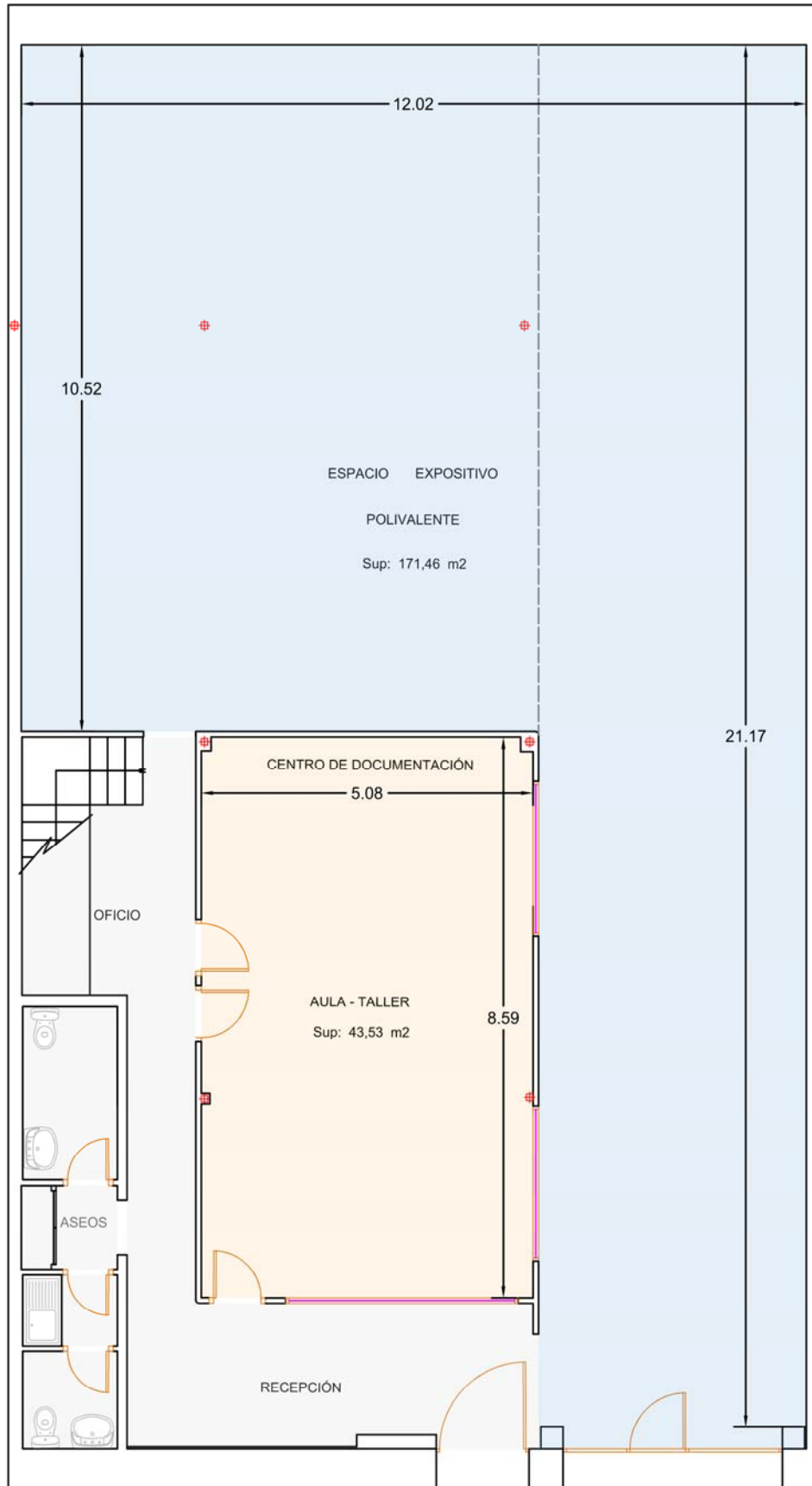
PLANTA BAJA
