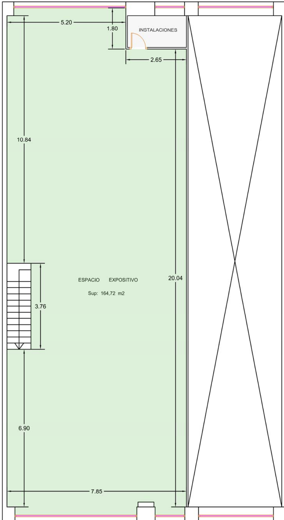
PLANTA ALTA
